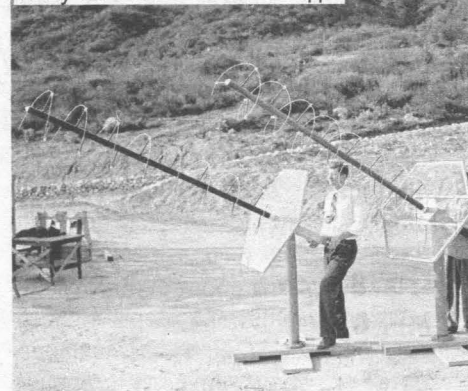
Испытание макетов акустических излучателей в 1950-е годы
